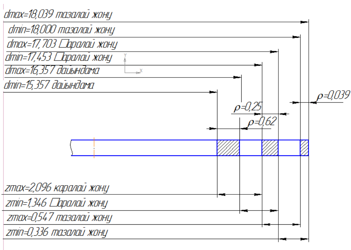
2.6.1.-Сурет-Тесік үшін \emptyset 18f8^{+0,039} әдіп және шаптаманың орналасу схемасы.
