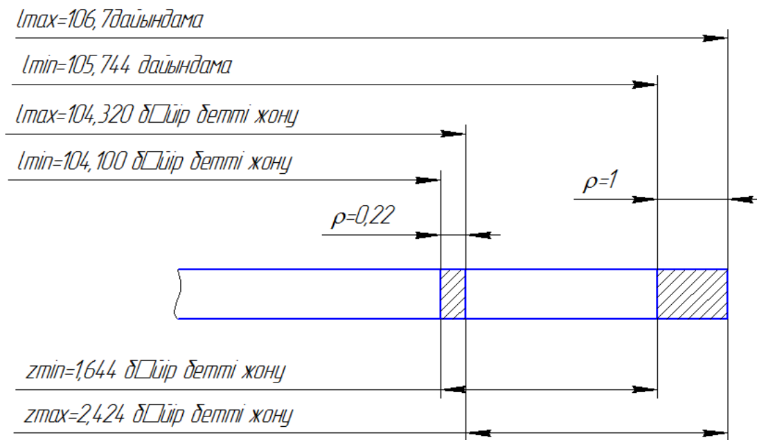
Сурет 2.6.2-Сыртқы бөлігі 108 ^{-0,25} мм үшін әдіп және шақтаманың схемасы
